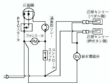
【配線図】
