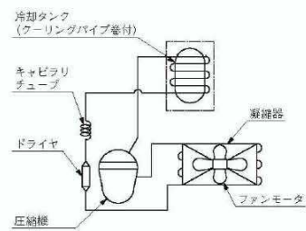
【冷凍サイクル図】
