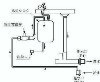
【水回路図】
