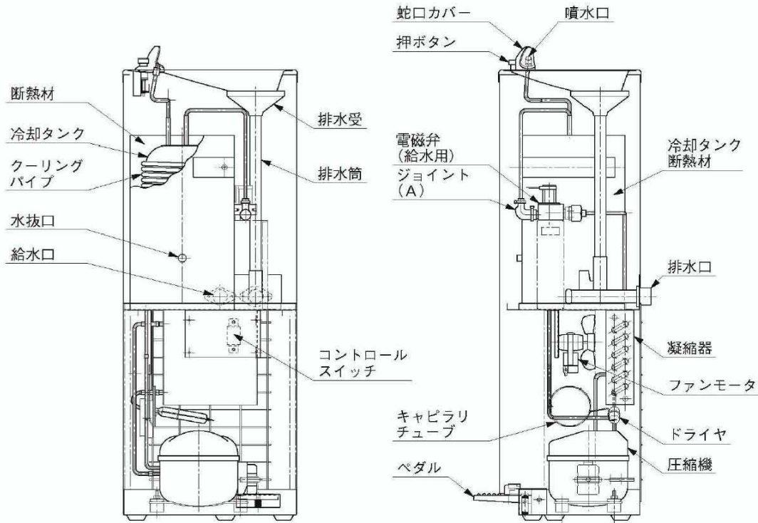
【構造図】
