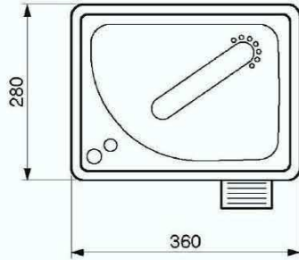
【外形図】
